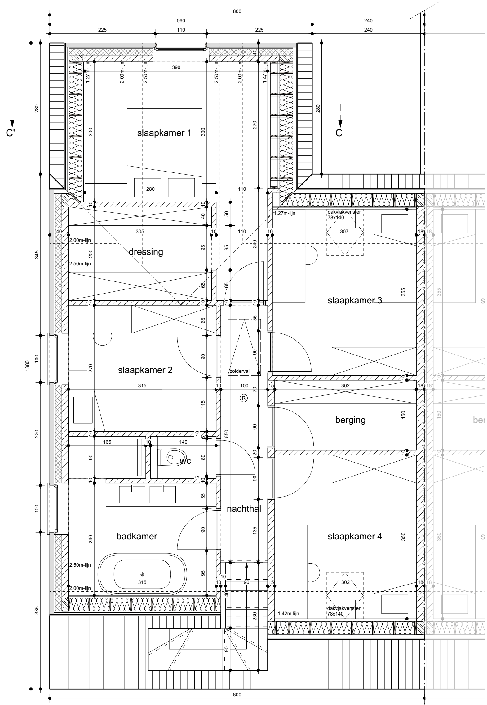
Verdieping LOT B schaal 1/50
